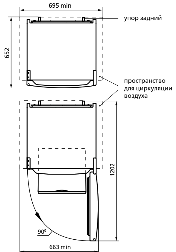
Рисунок 2 – Холодильник (вид сверху)
