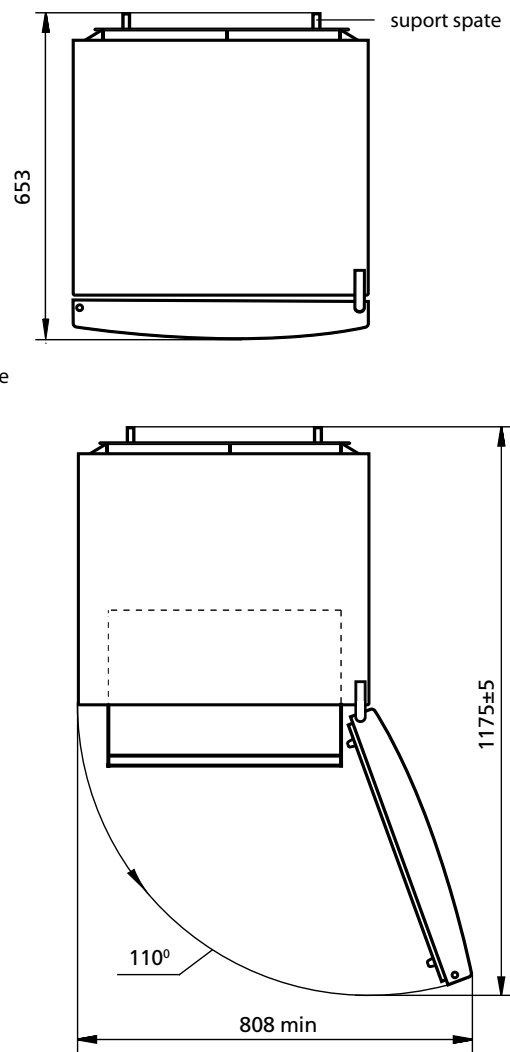
Desen 2 – Frigider (imaginea de sus)
