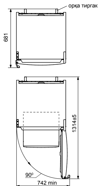
2-расм — Совутқич (уст қисми) кўриниши
