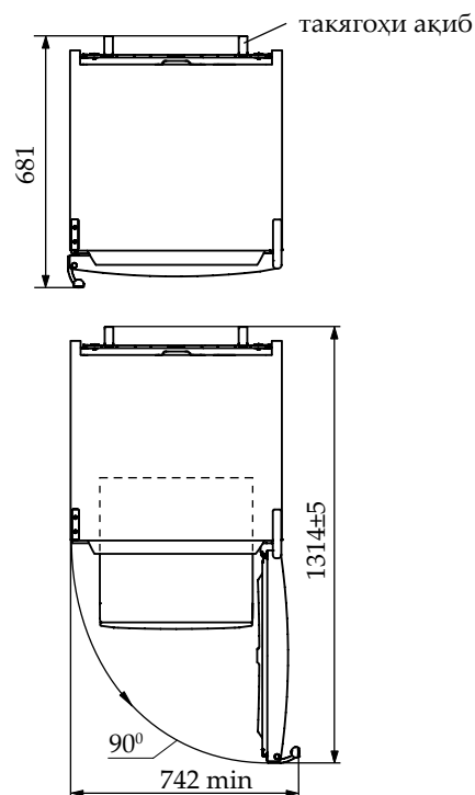
Расми 2 — Яхдон (намуди он аз боло)
