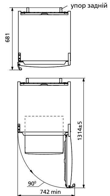
Рисунок 2 — Холодильник (вигляд зверху)
