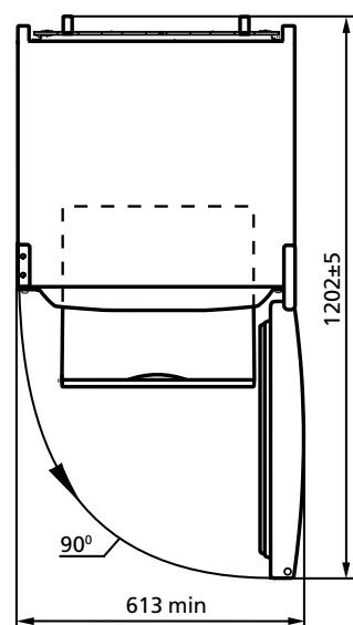
2-сүрөт – Муздаткыч (үстүнөн көрүнүшү)
