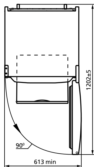
2 Rasm – Sovutgich (ust tomondan ko'rinish)
