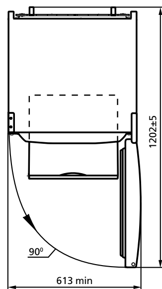
Imagine 2 – Frigider (vedere de sus)
