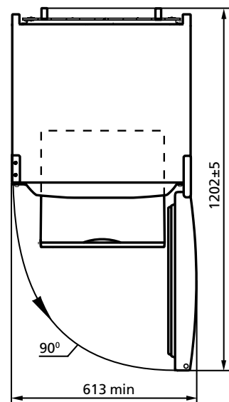
Rəsim 2 – Soyuducu (üstədən görünüşü)
