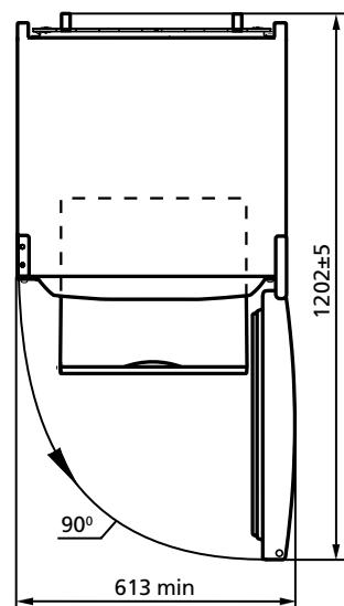
2 сурет – Тоңазытқыш (үстінен көрініс)
