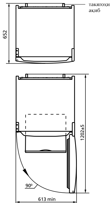
Расми 2 – Яхдон (намуди он аз боло)
