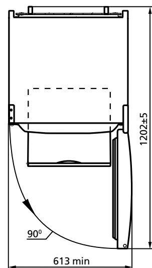
Рисунок 2 – Холодильник (вид зверху)
