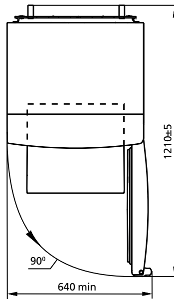
Şəkil 2 – Soyuducu (yuxarıdan görünüş)
