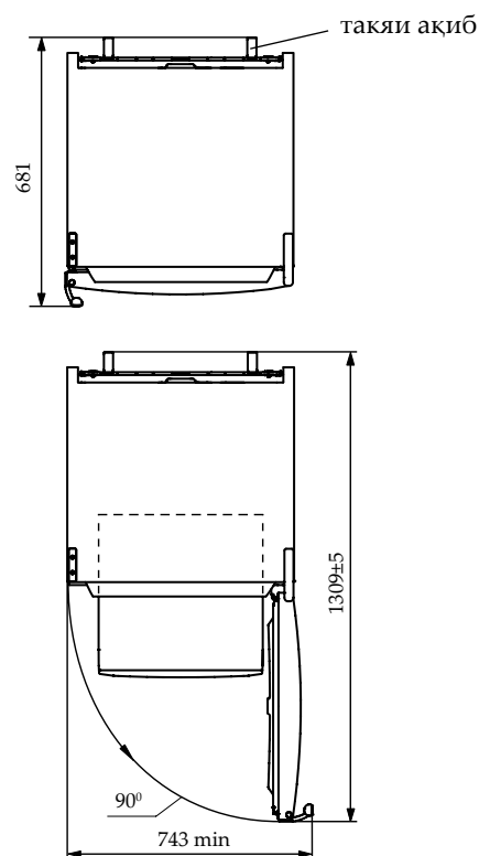
Расми 2 – Яхдон (намои болоӣ)
