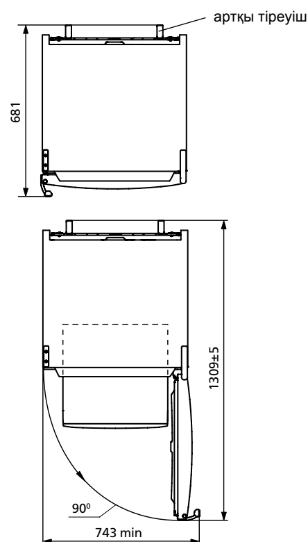
2 сурет – Тоңазытқыш (үстінен қарау)
