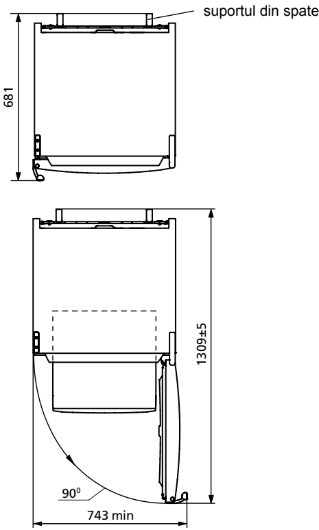
Figura 2 – Frigiderul (privire de sus)
