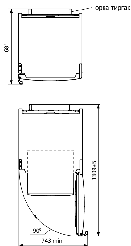
2-расм – Совуткич (юқоридан кўриниши)
