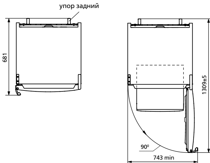
Рисунок 2 – Холодильник (вид сверху)
