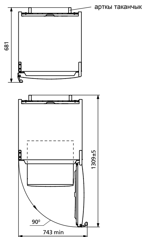
2-сүрөт – Муздаткыч (үстүнөн караганда)
