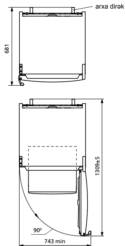
Şəkil 2 – Soyuducu (yuxarıdan görüntüsü)
