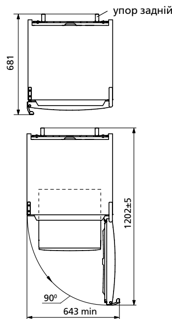
Рисунок 2 – Холодильник (вид зверху)
