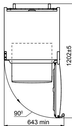
2-сурет – Тоңазытқыш (үстінен қарау)
