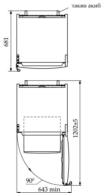
Расми 2 – Яхдон (намои болоӣ)
