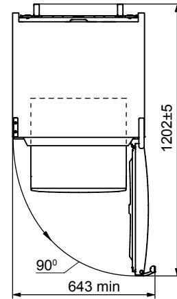
Şəkil 2 – Soyuducu (yuxarıdan görüntüsü)
