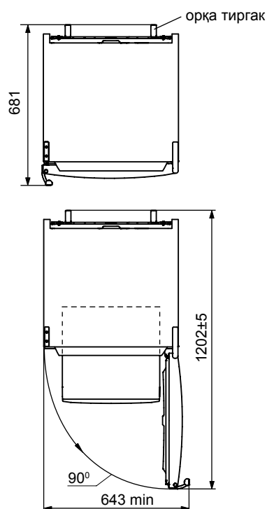
2-расм – Совуткич (юқоридан кўриниши)
