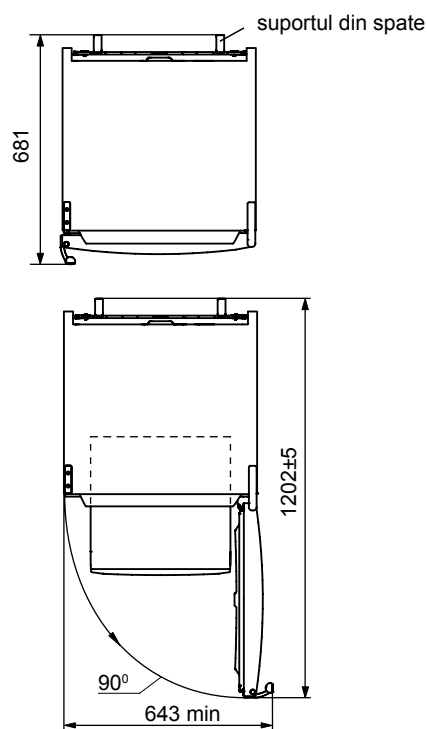
Figura 2 – Frigiderul (privire de sus)
