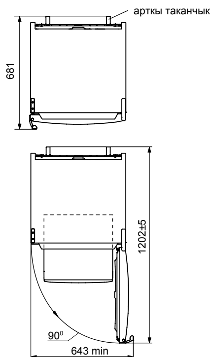
2-сүрөт – Муздаткыч (үстүнөн караганда)
