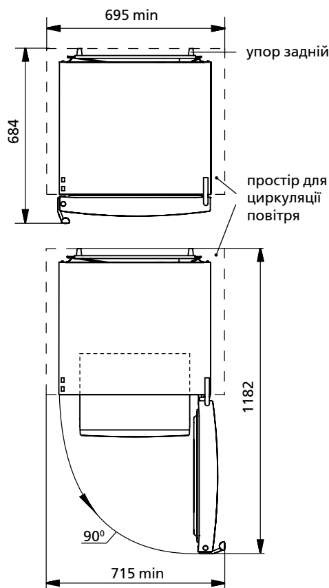
Рисунок 2 – Морозильник (вигляд зверху)
