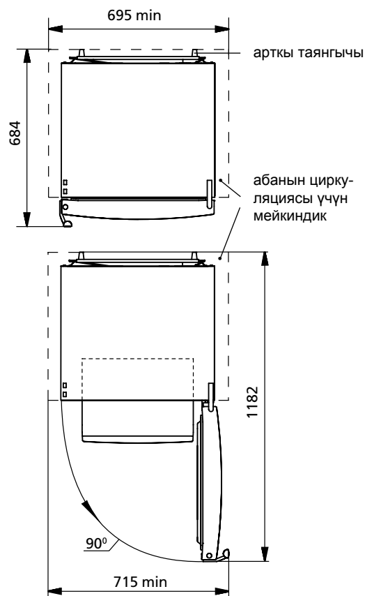
Сурот 2 – Тоңдургуч (устунон корсотулгон)
